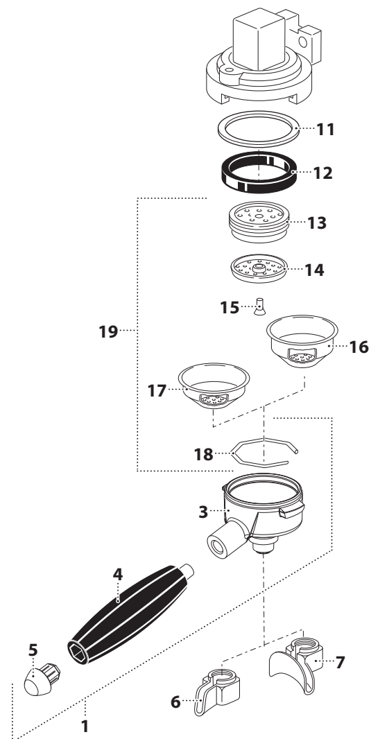
PORTAFILTRO PER CIALDA POD PORTAFILTER
